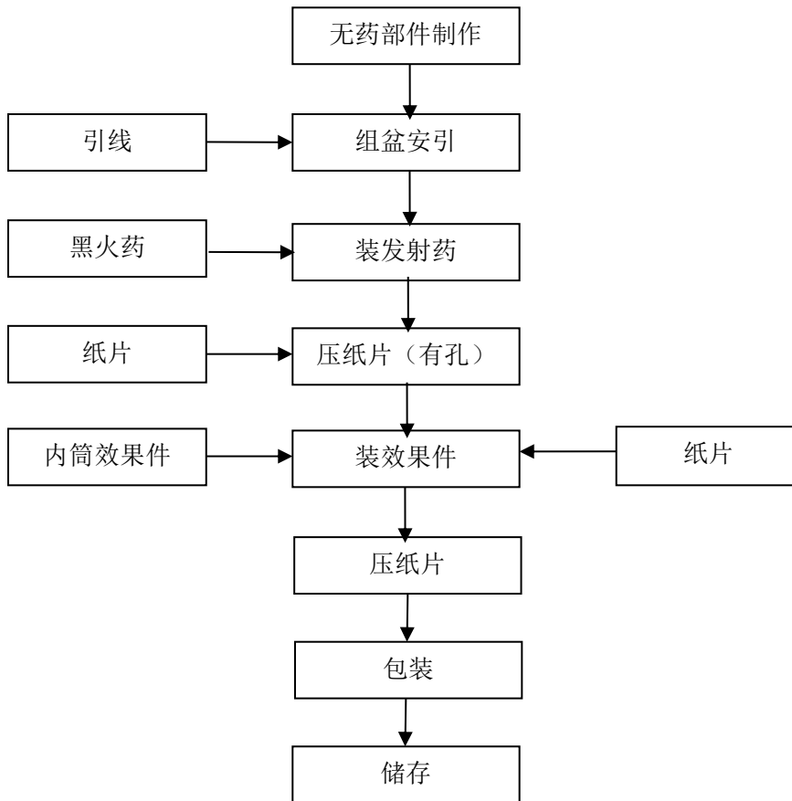
图 2.4-3 组合烟花生产工艺流程图
