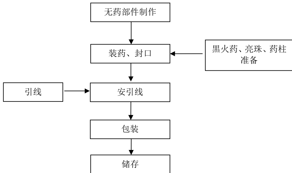
图 2.4-4 喷花类产品生产工艺流程图
