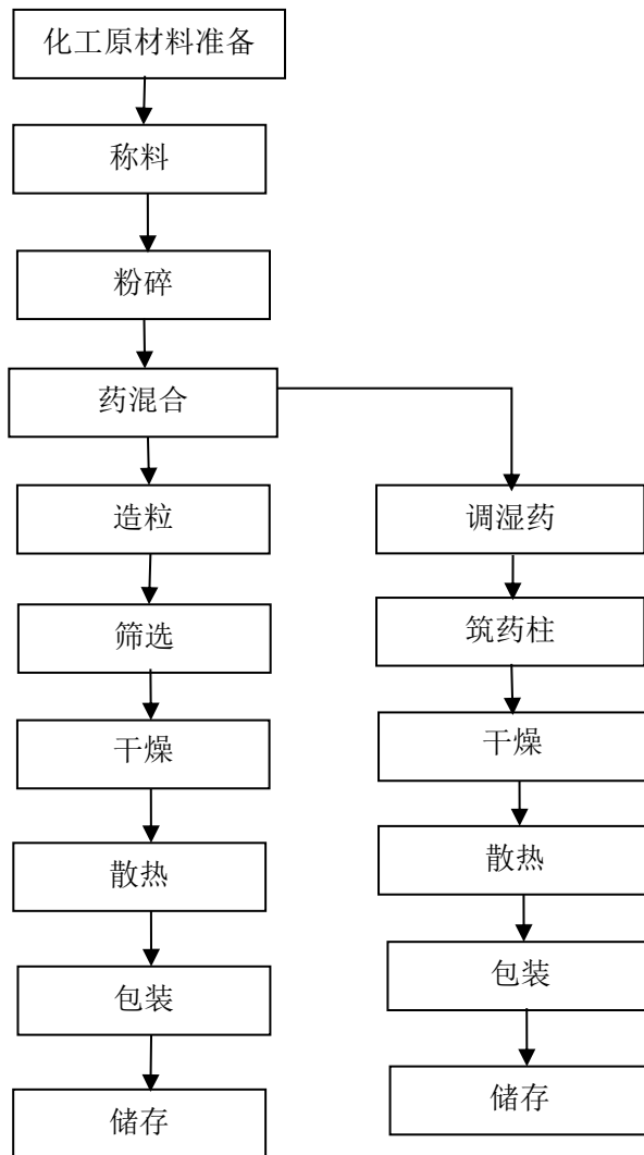
图 2.4-1 亮珠、药柱生产工艺流程图
