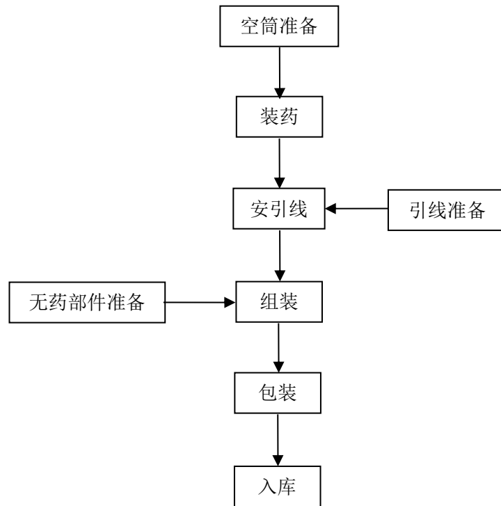
图 2-4-5 玩具类（玩具造型）生产工艺流程图
