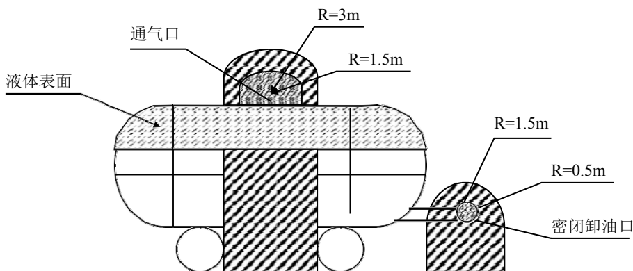
图 3-2 汽油油罐车爆炸危险区域划分
