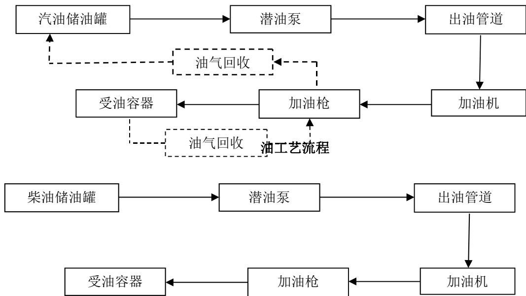
图 2-7 柴油加油工艺流程
