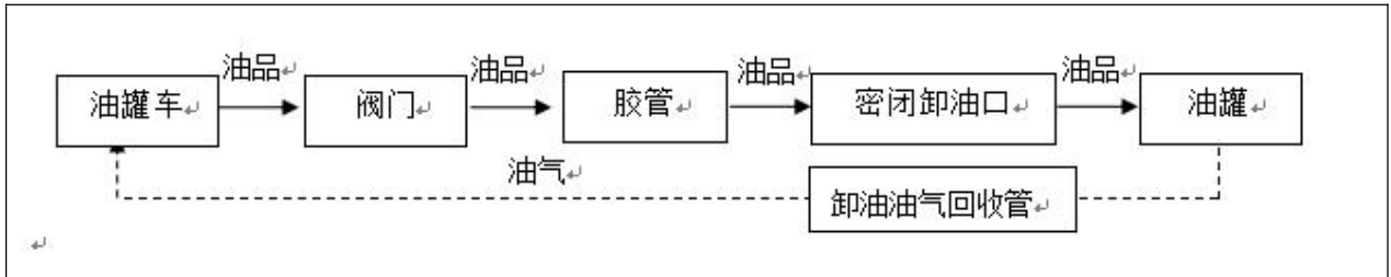
图 2.6-3 汽油卸油工艺流程图
