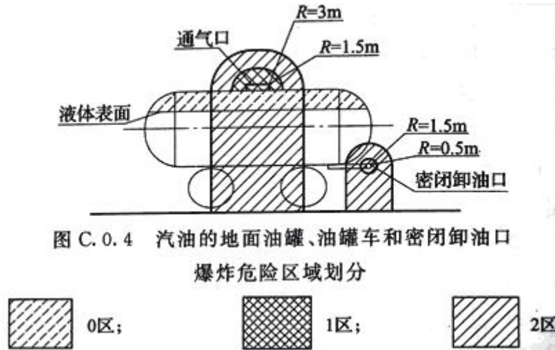
图 3.12-3 油罐车卸汽油爆炸危险区域
