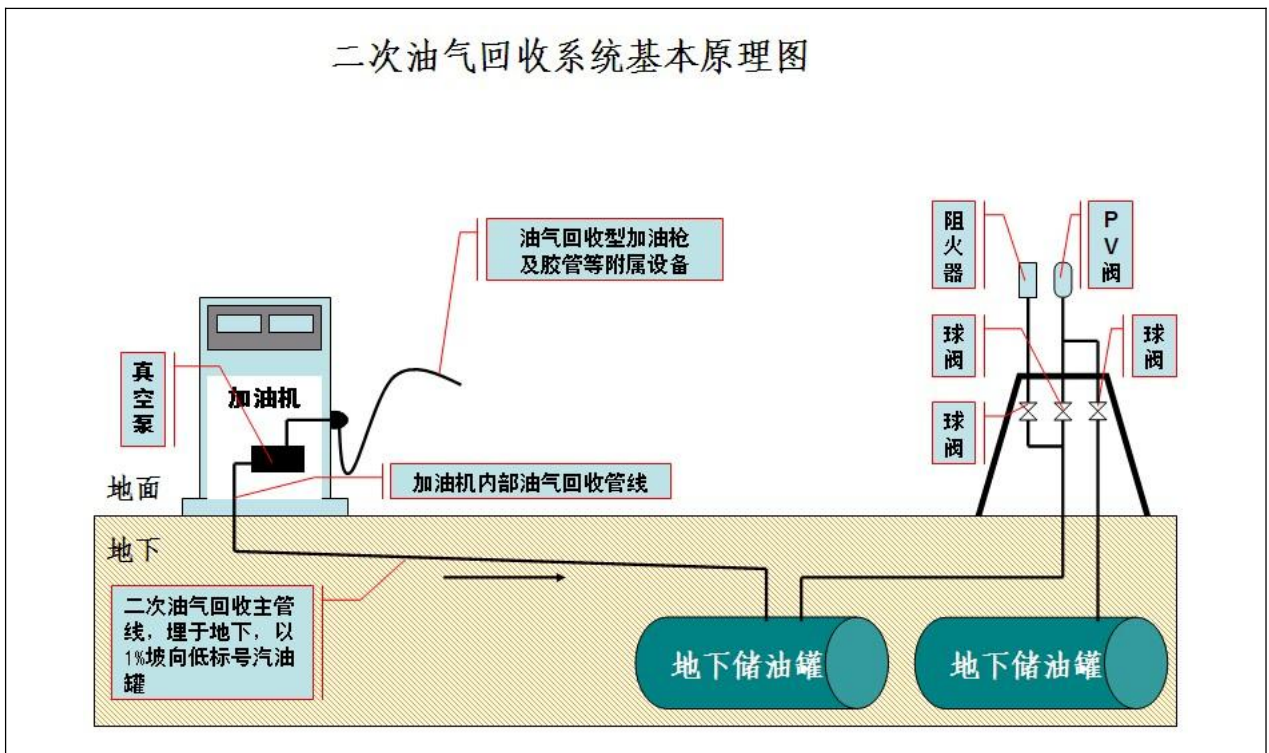
图 2.6-5 二次油气回收系统基本原理图
