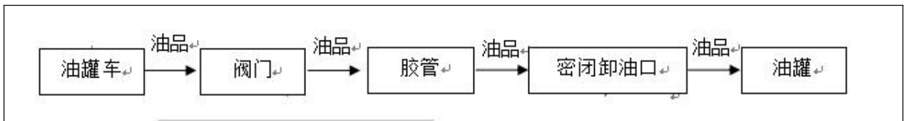
图 2.6-4 柴油卸油工艺流程图
