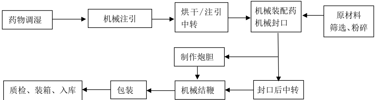
图 2-1：爆竹生产（注引）工艺流程图
