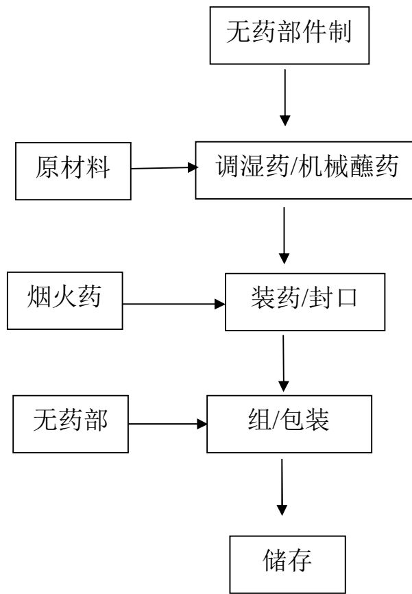
图 2.3-4 玩具类（线香型/晨光花）生产工艺流程图
