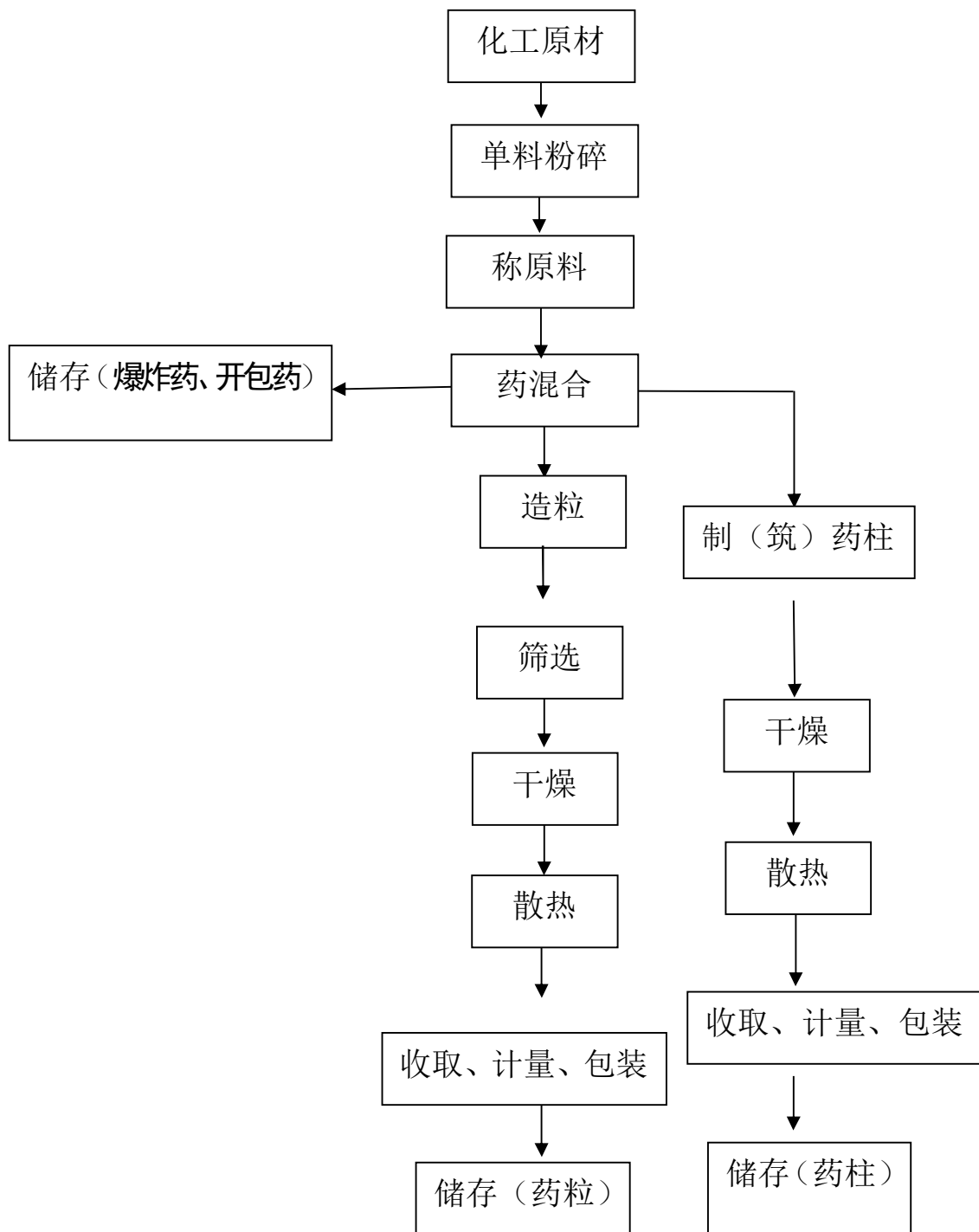
图 2.3-1 药物裸药效果件生产工艺流程图（药粒、药柱）
