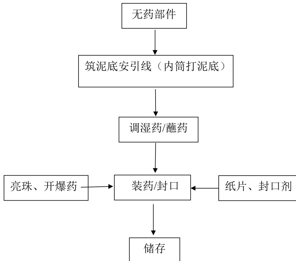
图 2.3-2 效果内筒生产工艺流程
