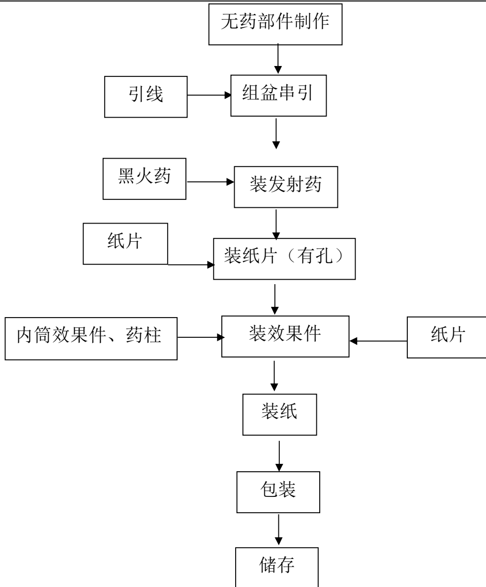
图 2.3-3 组合烟花生产工艺流程图
