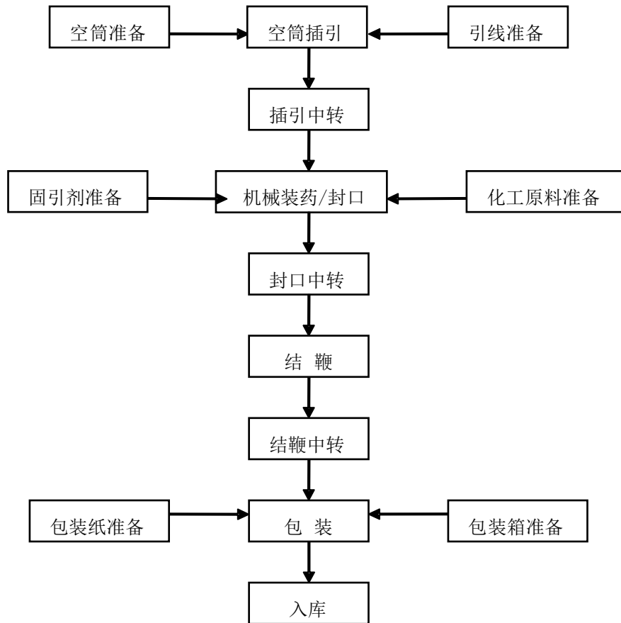
图 2-4-1 爆竹类产品生产工艺流程图
