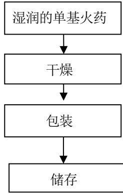
图 2-4-1 单基火药生产工艺流程图
