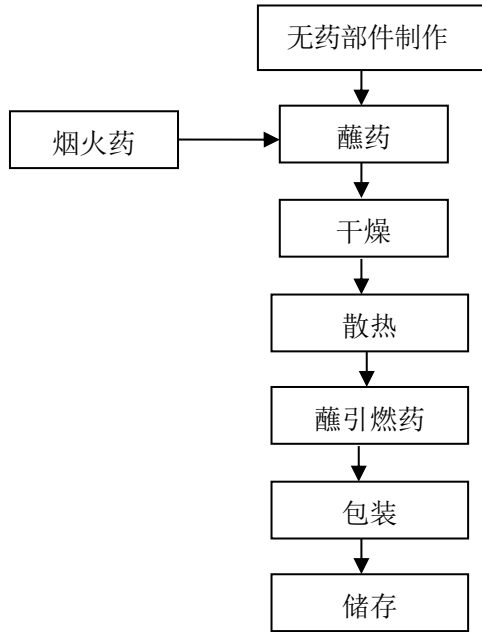
图 2-4-2 玩具类（线香型/涂敷型）生产工艺流程图
