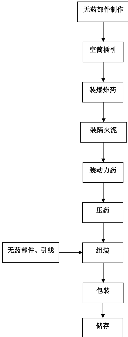
图 2-4-1 升空类（小型火箭）生产流程图
