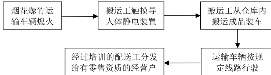
图 2-2-2-2 烟花爆竹出库工艺流程示意图
