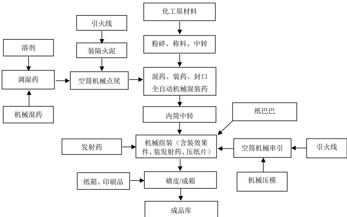
图2.3-1 组合烟花类（不含亮珠）机械组装生产工艺流程图
