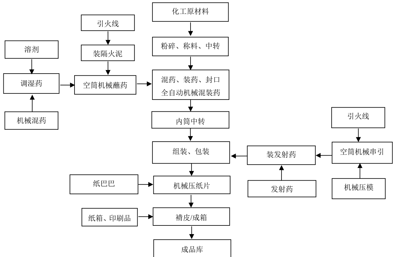
图2.3-2 组合烟花类（不含亮珠）手工组装生产工艺流程图
