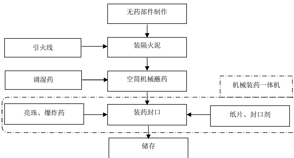
图 2-2: 效果内筒生产工艺流程图
