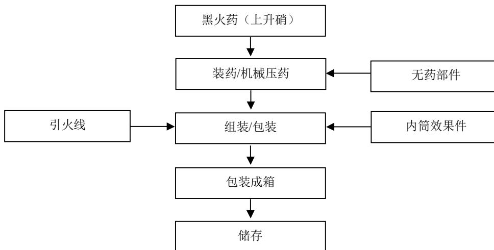
图 2-3: 升空类（火箭）产品生产工艺流程图
