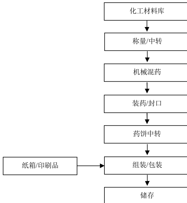
图 2-6: 玩具类（线香型）产品生产工艺流程图
