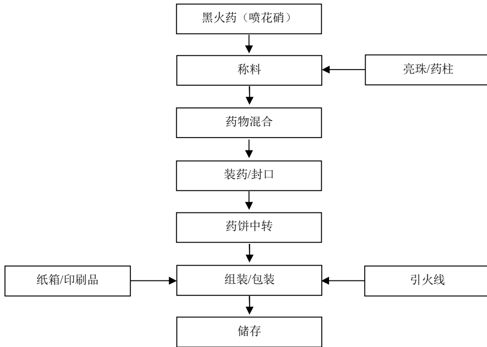
图 2-5: 喷花类产品生产工艺流程图
