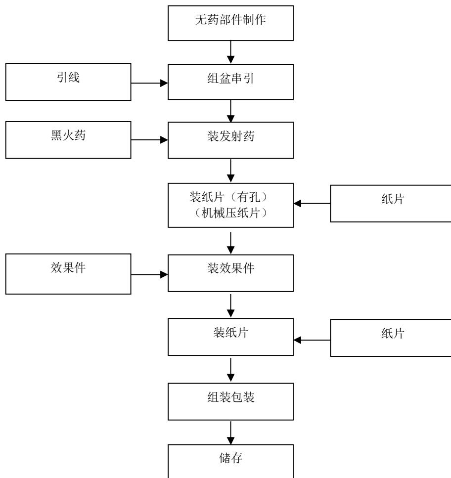
图 2-1：组合烟花生产工艺流程图
