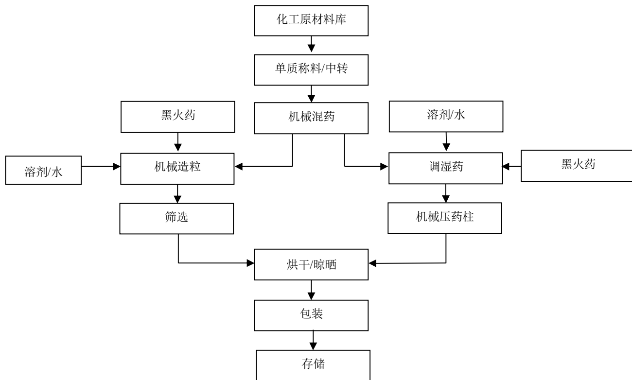
图 2-7：亮珠/药柱生产工艺流程图
