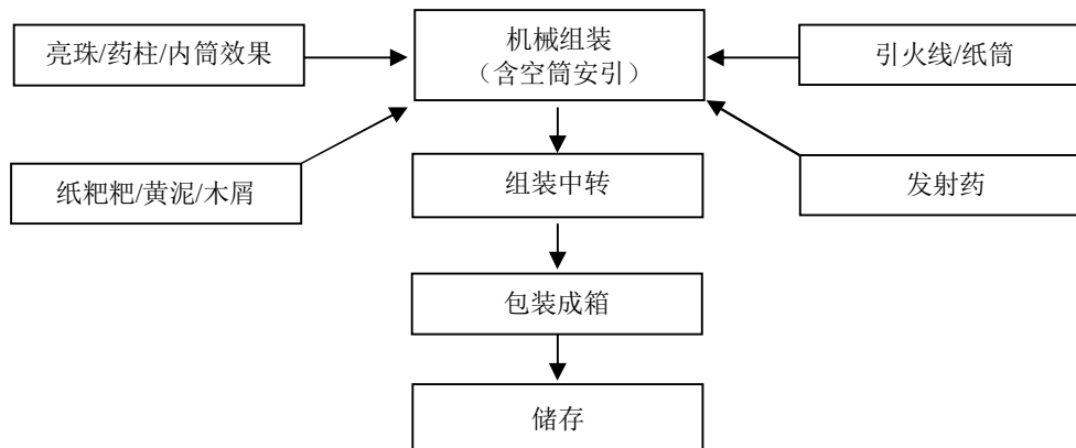
图 2-4: 吐珠类产品生产工艺流程图
